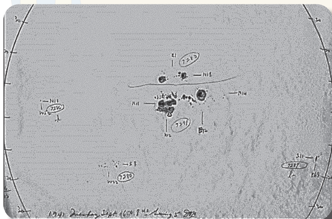
Le macchie solari osservate dal Mount Wilson Observatory, in California, il 16 settembre 1941 - © Carnegie Observatories
