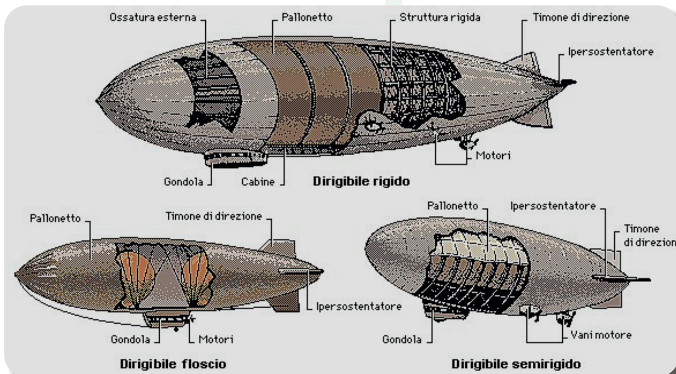
Tipologie di dirigibile - Fonte: dida.fausser.edu
